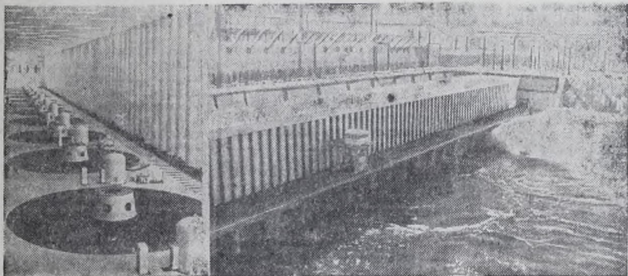
Асуанский гидроэнергетический комплекс — символ современного Египта. На снимках: машинный зал ГЭС; здание ГЭС.
