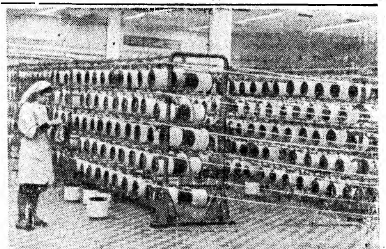
В этом цехе обрабатывается нить высокопрочного курского лавсана. Здесь ее собирают в жгуты для последующих операций. Минувший год для коллектива Курского завода синтетического волокна был годом больших трудовых побед. Переработано несколько миллионов килограммов полиэфирных лавсановых смол и получено лавсанового волокна значительно больше, чем предусматривалось планом. Фото О. Сизова.
