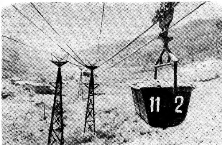
Канатно-подвесная дорога на мраморном карьере «Перевал», построенном ангарскими строителями. Карьер снабжает сырьем ангарский цементный завод.
