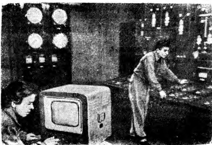
Луганская область. В цехе производства аммиачной селитры Лисичанского химического комбината действует опытная промышленная телевизионная установка с дистанционным управлением передающей камеры.
