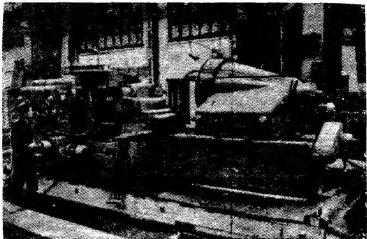
Коллектив сборочного цеха Краматорского завода тяжелого станкостроения изготовил для Республики Индии колесотоккарный станок, оборудованный гидравлическими суппортами. Станок собрала передовая бригада слесарей, возглавляемая И. Н. Сирихом. На снимке: колесотоккарный станок, подготовляемый к отправке в Индию. Фотохроника ТАСС.
