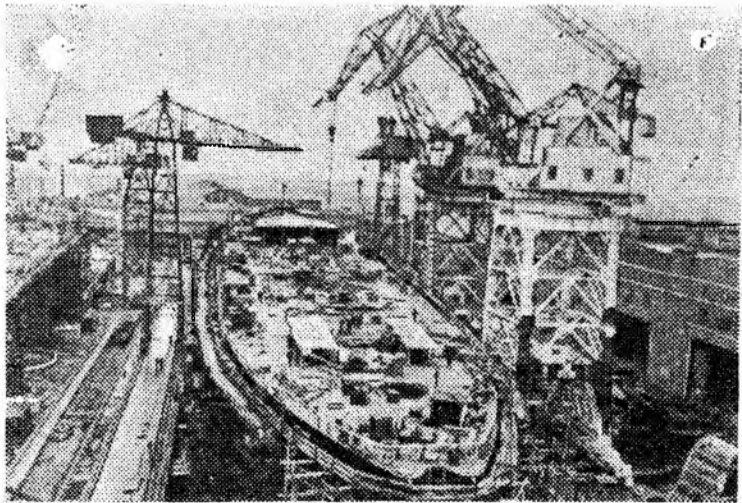
Ленинград. На строительстве атомного ледокола «Ленин». На снимке: общий вид строительства ледокола.
