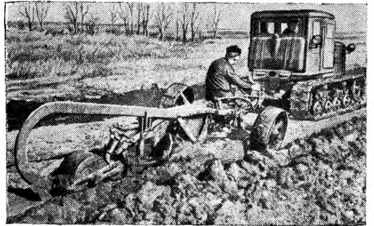
Черниговская область. Механизаторы Нежинской лугомелиоративной станции имени Н. С. Хрущева, став на трудовую вахту в честь 300-летия воссоединения Украины с Россией, обязались освоить в этом году свыше трех тысяч гектаров болотных земель. План первого квартала по всем видам работ станция выполнила на 146 процентов.
