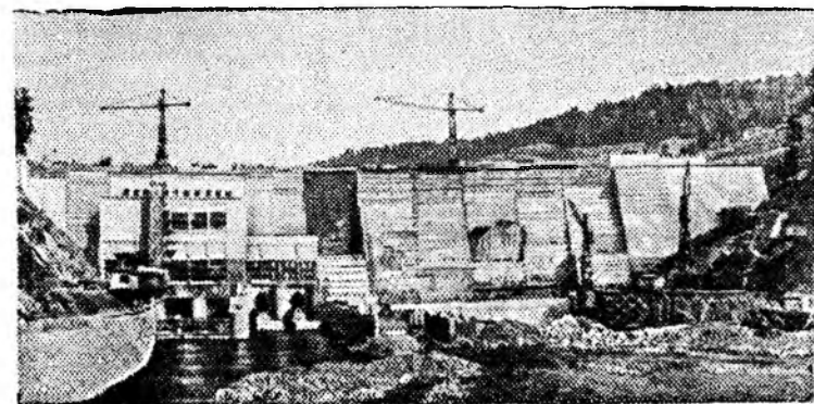
Чехословацкая республика. Общий вид строящейся Вирской плотины. Фото Чехословацкого телеграфического агентства.
