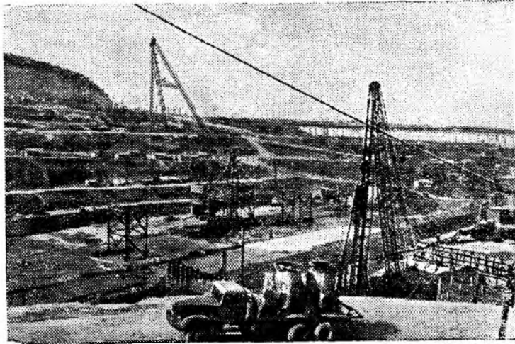
Куйбышевгидрострой. Общий вид работ в районе строительства котлована под здание ГЭС.
