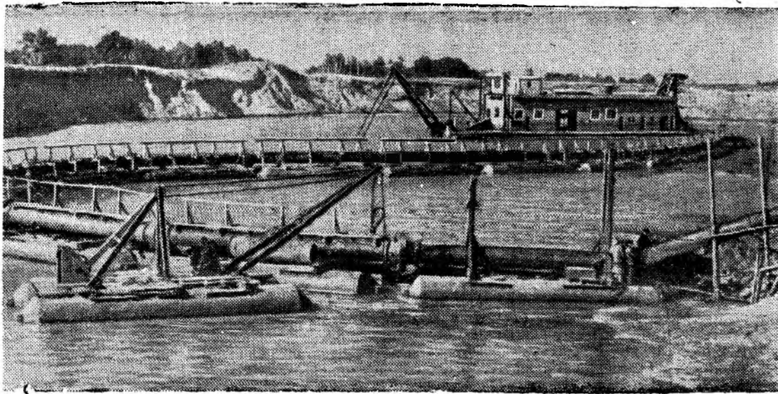
Сталинградгидрострой. Комсомольско-молодежный земснаряд 501 производит выемку грунта и намыв дамбы на трассе нижнего подходного канала к шлюзу со стороны Волги.
