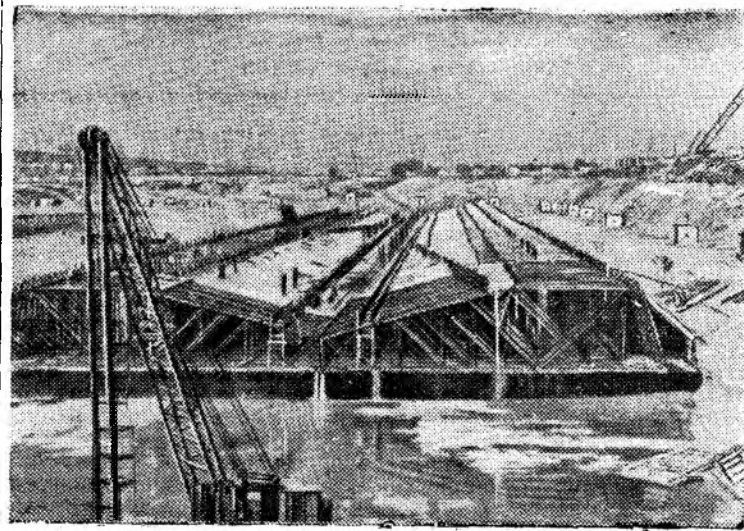
Куйбышевгидрострой. На строительстве камер нижнего судоходного шлюза идет монтаж металлоконструкций и укладка бетона. На снимке: общий вид бетонизируемых блоков днища камер нижнего судоходного шлюза.
