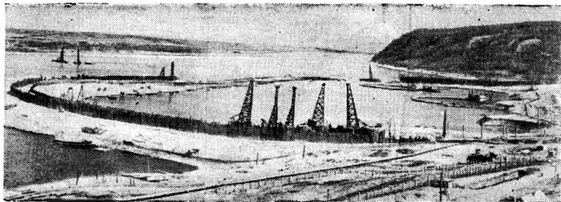
КУЙБЫШЕВГИДРОСТРОЙ. Строительство котлована под здание гидроэлектростанции. Фото Н. Финикова.
