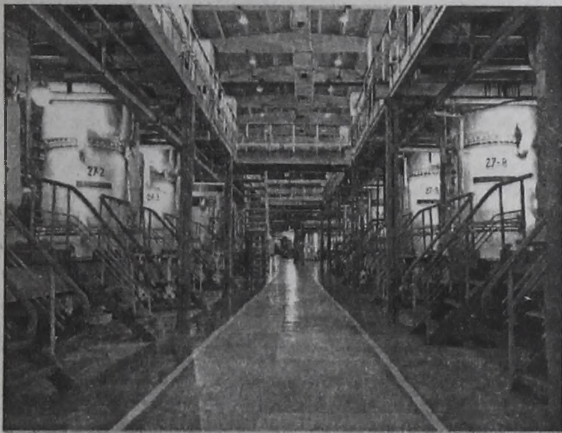
Производство гексафторида урана на сублиматном заводе.
