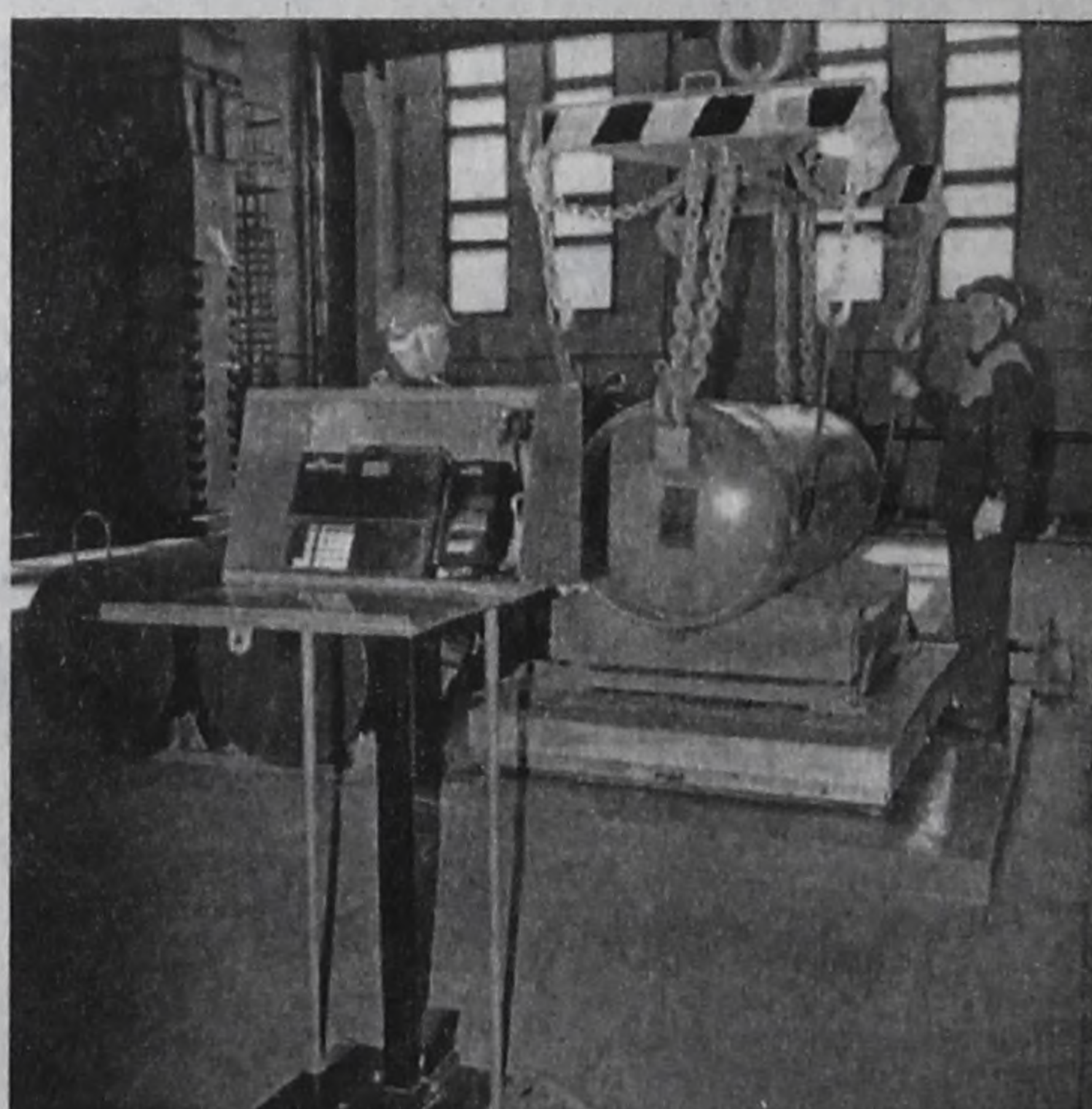
Взвешивание контейнера с гексафторидом урана.
