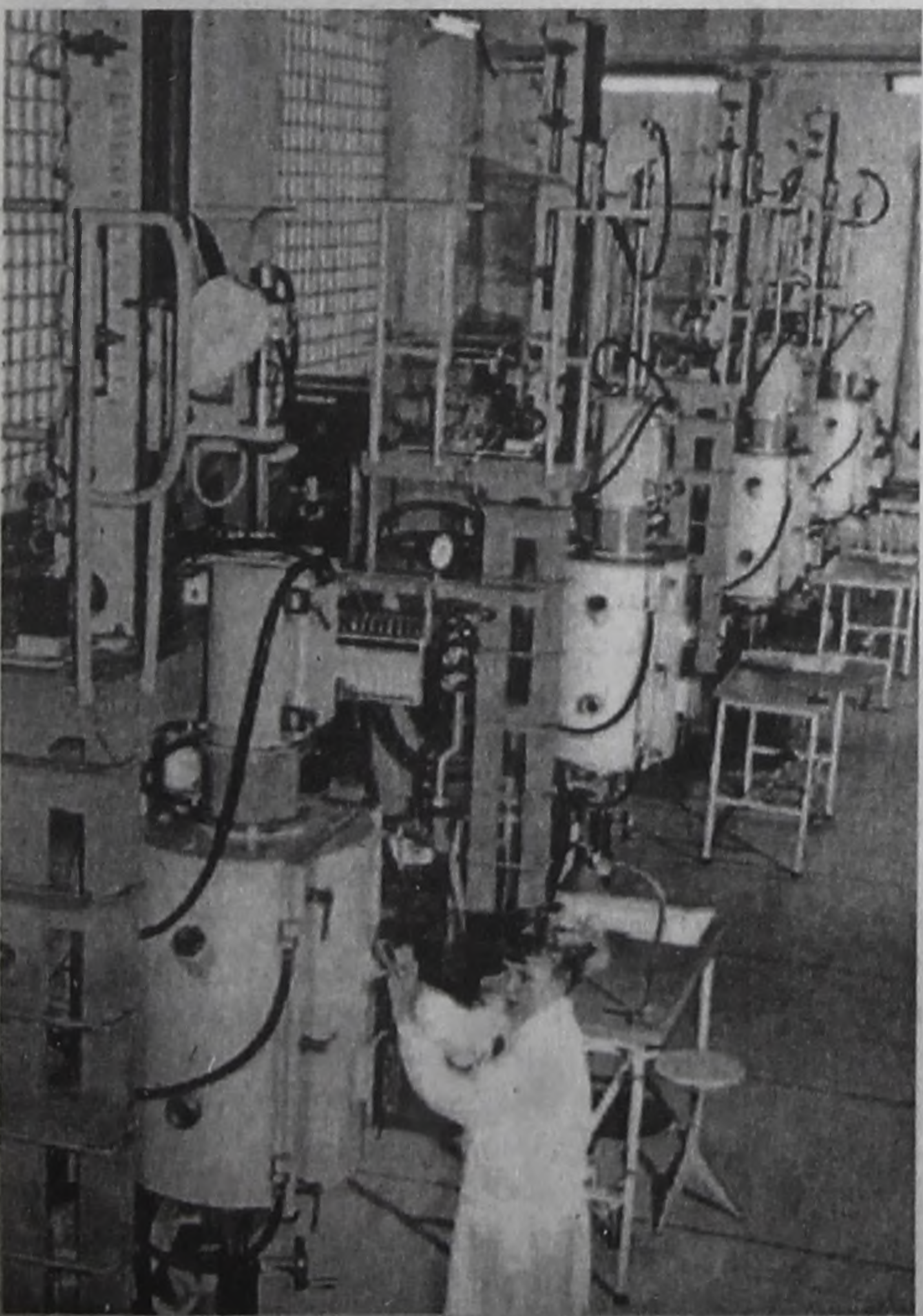
Зал установок выращивания кристаллов.
