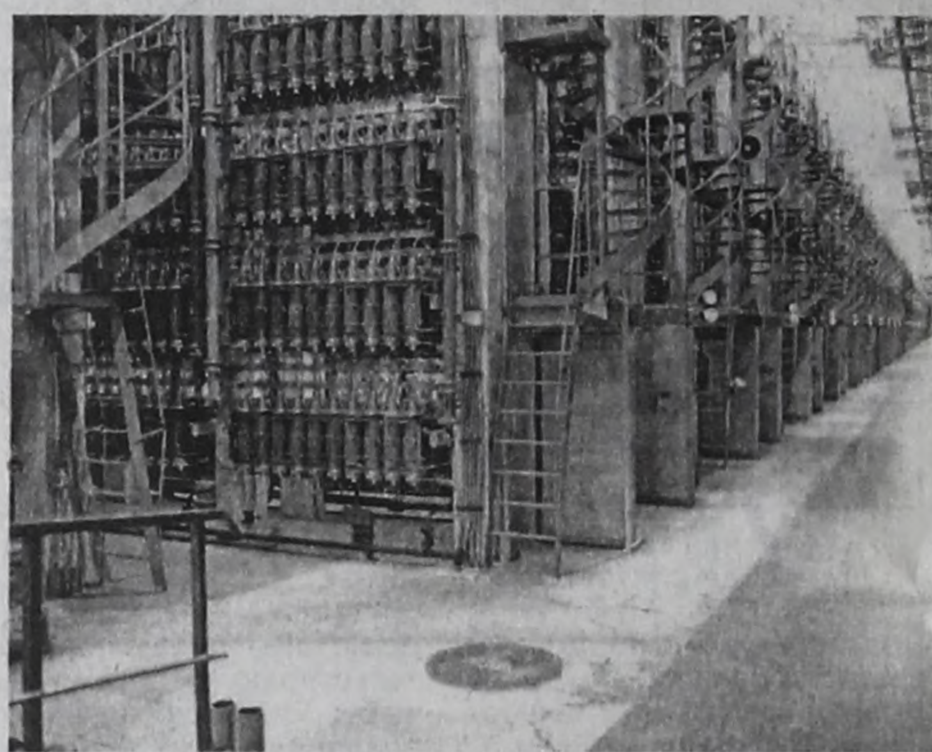
Завод по обогащению урана. Машинный зал.
