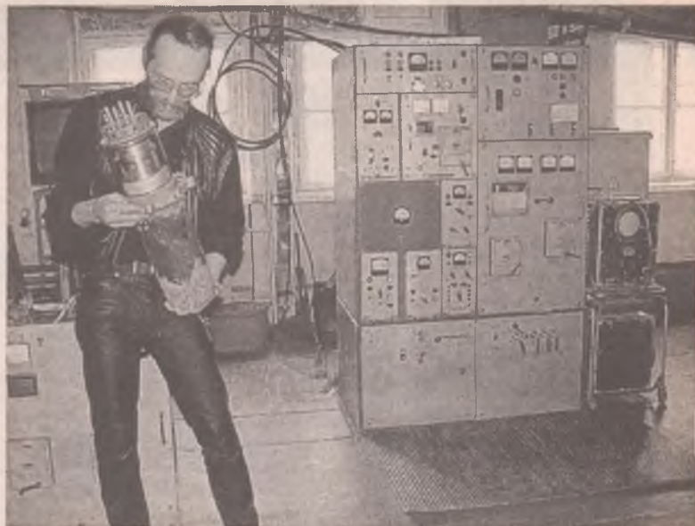
"Сердце" передатчика - анодная лампа.
