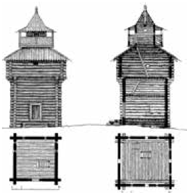
• Схема Бельской башни
