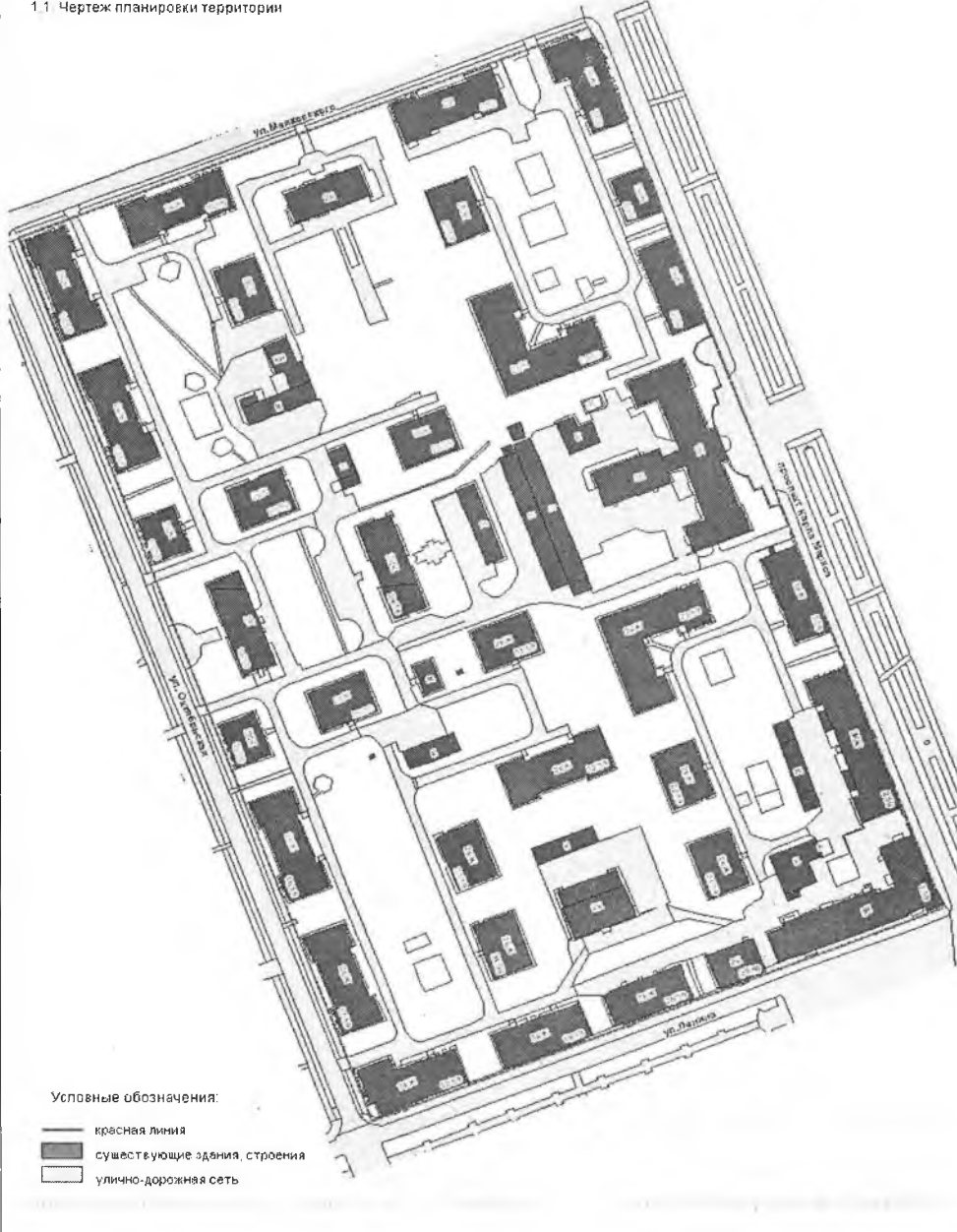
1.1. Чертеж планировки территории
