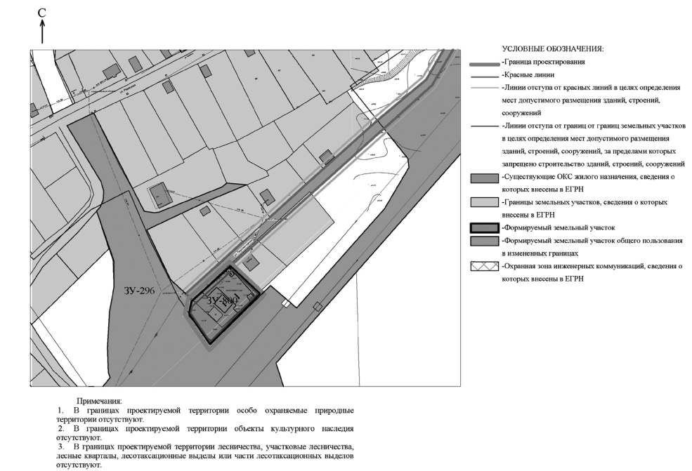
Фрагмент чертежа межевания территории (материалы по обоснованию)
