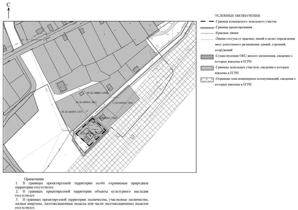
Фрагмент чертежа межевания территории (материалы по обоснованию)
