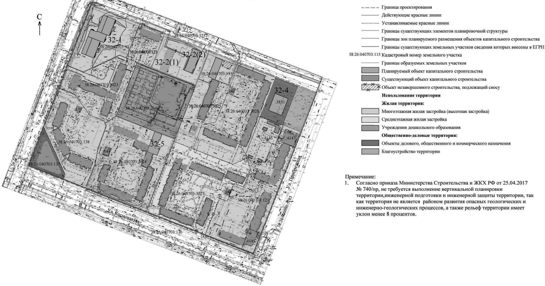
Схема вертикальной планировки территории, инженерной подготовки и инженерной защиты территории
