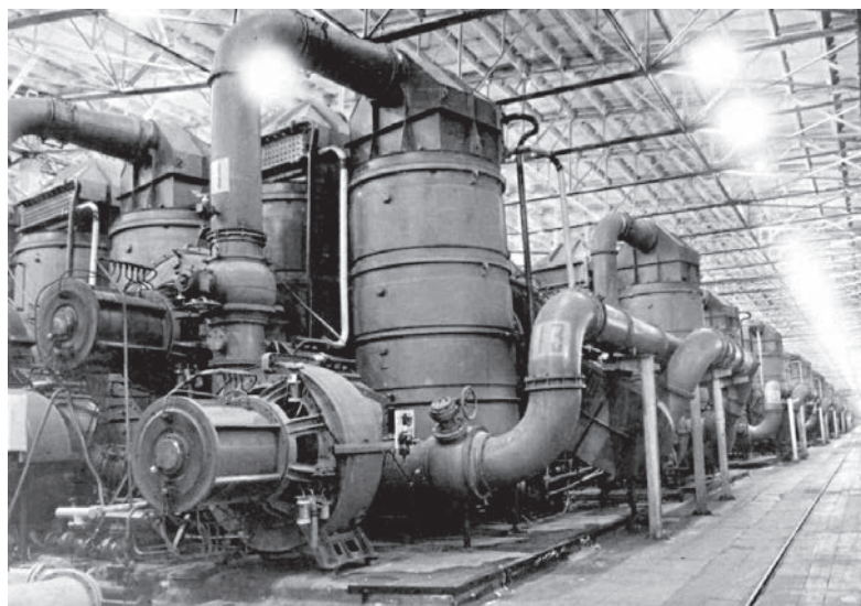
Так было, когда для обогащения урана использовали газодиффузионные установки
