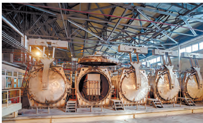
Автоклавы, в которых происходит изотермическая обработка продукции паром
