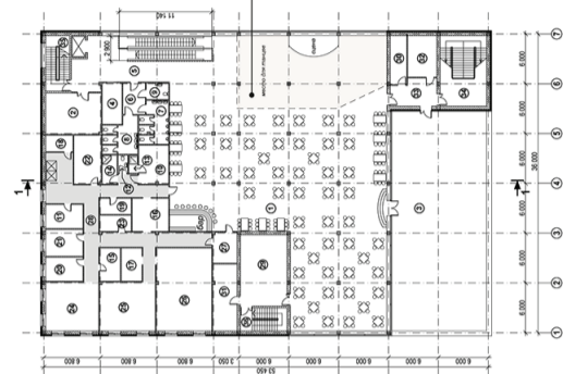
План на отк. 13,050
