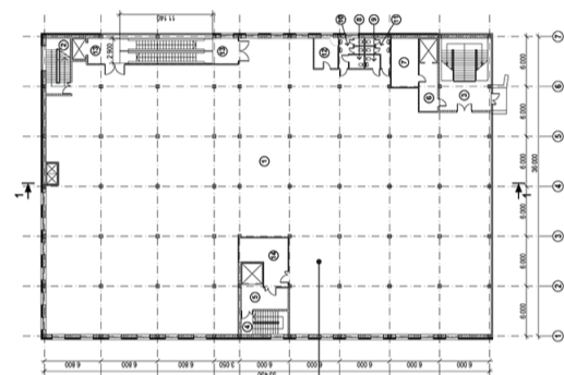
План на отк. 8,550
