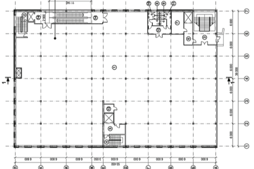
План на отк. 4,050
