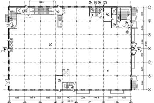
План на отк. 0,000
