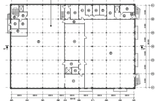
План на отк. -3,250
