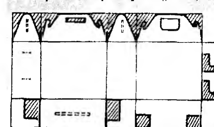
Рис. в. Чертеж.
