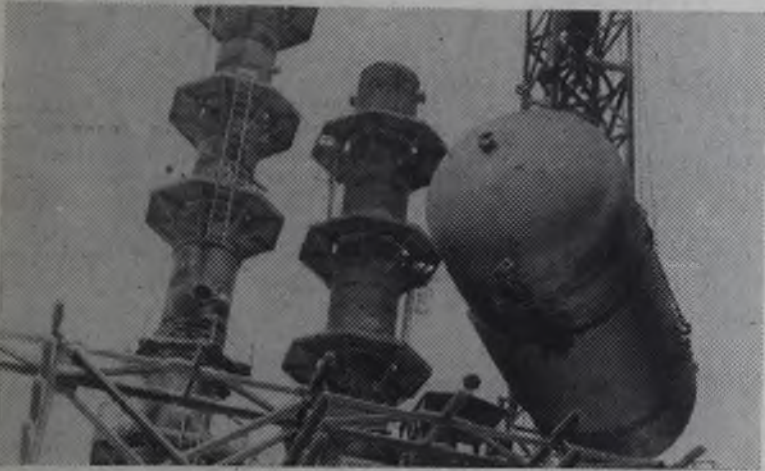
АНГАРСК. Этилбензол АНХК: идет монтаж оборудования.
