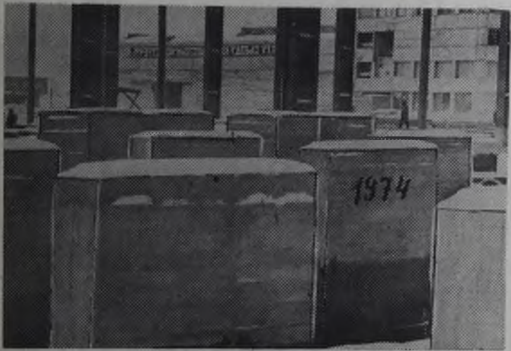
ЗИМА. Цех электролиза электрохимкомбината: фундаменты без оборудования.
