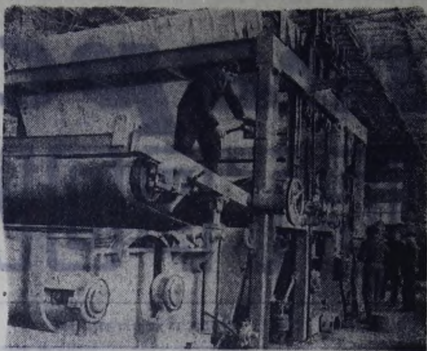
Опытная трубоформовочная машина «АТМ-4м» для производства асбоцементных труб малых диаметров изготовлена на могилевском заводе «Строммашина» имени 50-летия Великого Октября. Производительность ее на 20 процентов выше выпускаемой «АТМ-3». На ней будут изготавливать не трех-, а четырехметровые трубы. Обслуживают машину всего два человека — оператор и его помощник.
