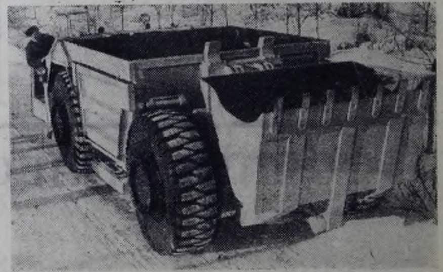
Свердловск. Эта машина предназначена для загрузки и транспортировки горной массы в подземных условиях при проведении горных выработок. Ее грузоподъемность 15 тонн, скорость движения до 30 километров в час, емкость кузова — 6 кубометров, ковша — 1,5 кубометра.
