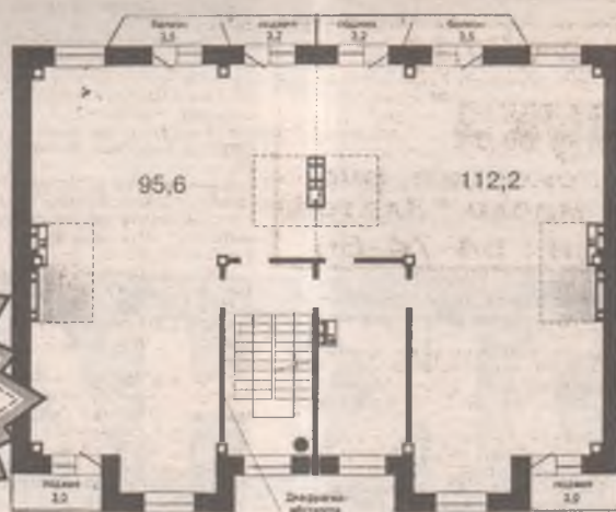
Типовой этаж блоксекции с основными стенами
