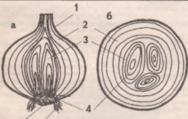
Луковица: а - продольный разрез; б - поперечный разрез; 1 - сухая покровная чешуя; 2 - открытые сочные чешуи; 3 - закрытые сочные чешуи; 4 - зачатки; 5 - донце; 6 - «пятка»
