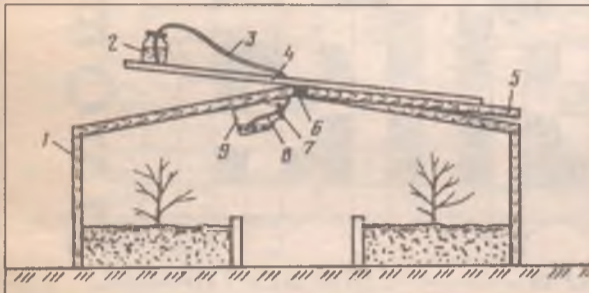
1 — каркас теплицы, 2 — стеклянная банка, вместимостью 1 л, с крышкой, 3 — гибкая трубка, 4 — рычаг, 5 — рама форточки, 6 — шарнир, 7 — крышка, 8 — металлическая трубка, 9 — стеклянная банка.
